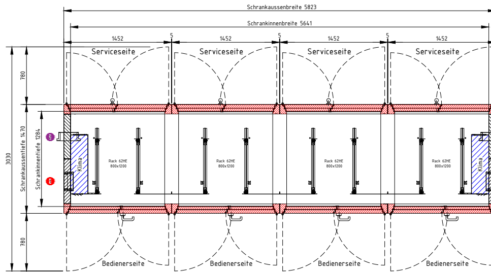
A-A ( 1 : 25 )
