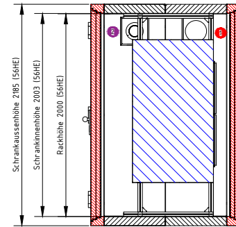
B-B ( 1 : 25 )
