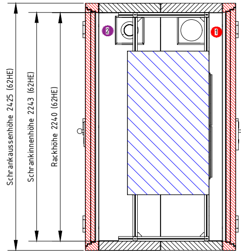
B-B ( 1 : 25 )
