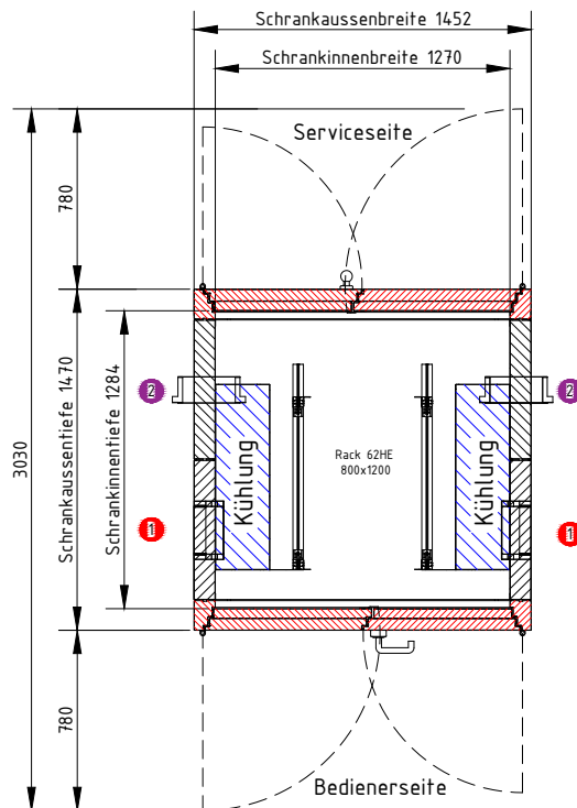
A-A ( 1 : 25 )
