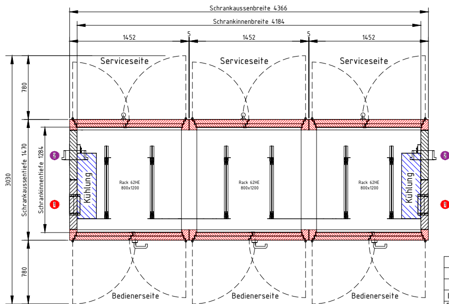
A-A ( 1 : 25 )
