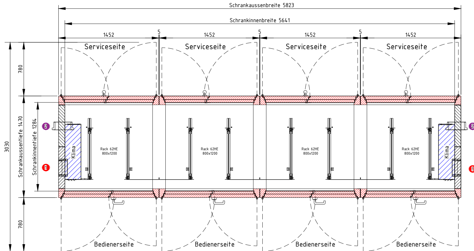
A-A ( 1 : 25 )
